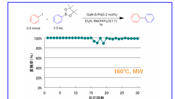
図2 鈴木-宮浦反応での繰り返し使用
